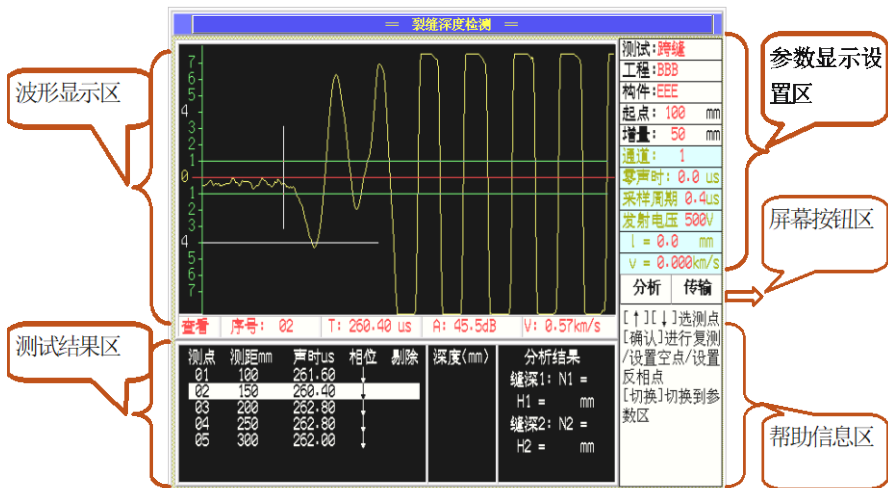
图 4.1 测缝主界面
