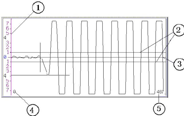
图 2.15 波形显示区
