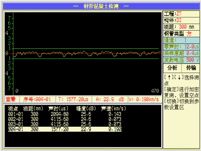
图 7.7 方管测试界面
