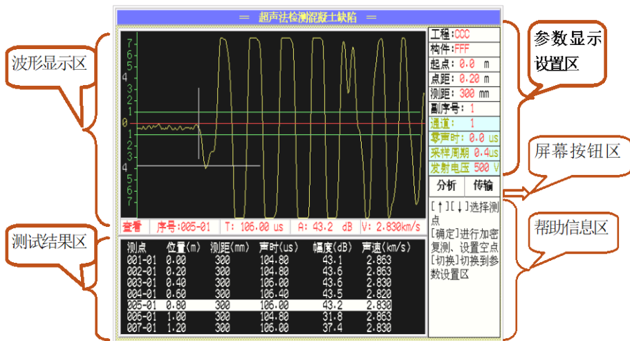
图 3.1 测缺主界面
