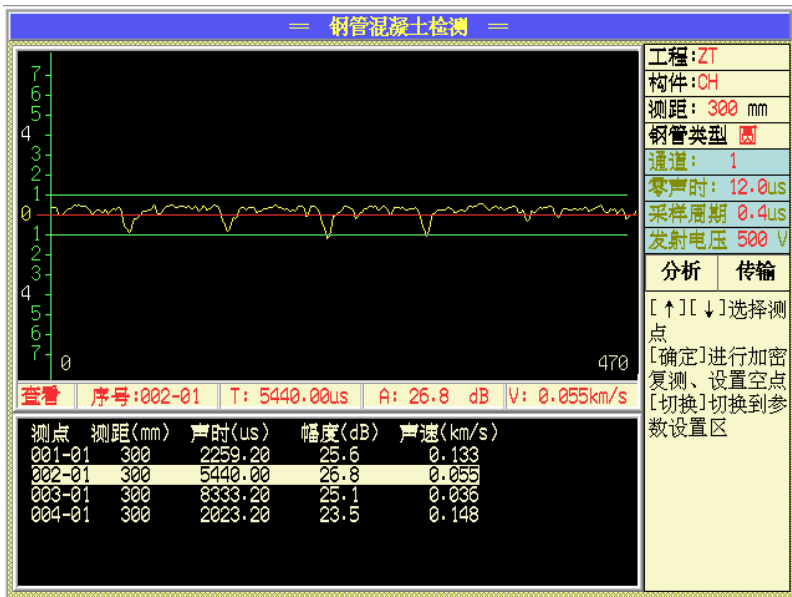
图 7.8 圆管测试界面
