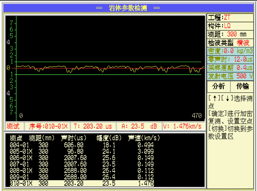
图 6.8 横波测试界面
