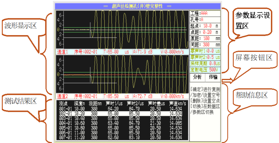
图 8.1 测井主界面
