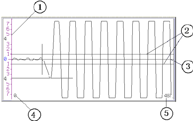
图 7.12 波形显示区
