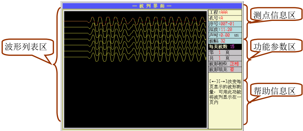
图 8.17 波列界面
