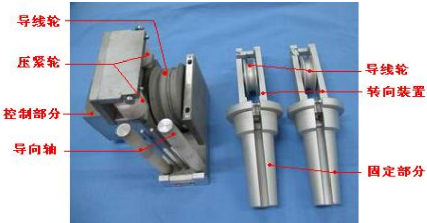
图 2.1 提升装置
