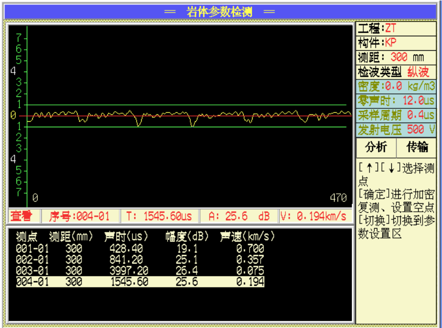
图 6.7 纵波测试界面
