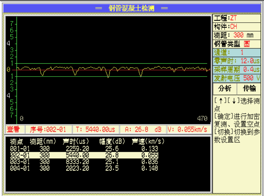
图 7.1 钢管混凝土测试主界面
