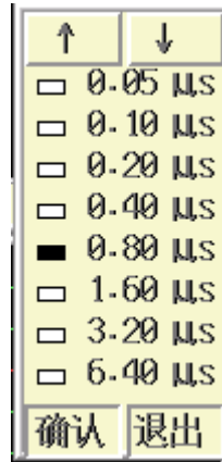
图 2.12 选择采样周期
