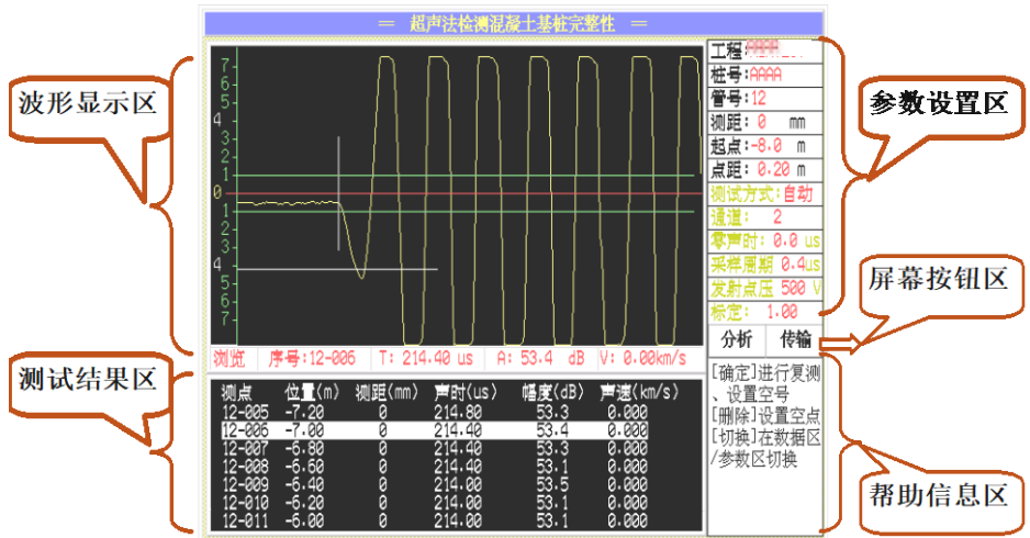
图 2.1 测桩主界面
