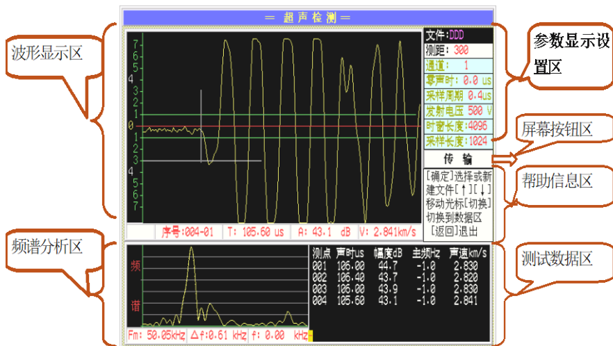
图 9.1 超声检测主界面
