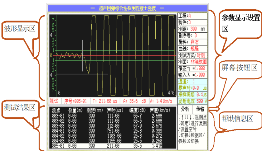
图 5.1 测强主界面
