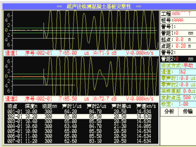
图 2.10 双通道测试界面
