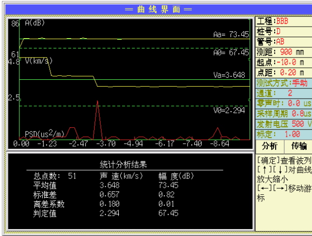
图 2.24 结果曲线界面
