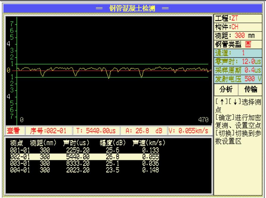
图 7.8 圆管测试界面
