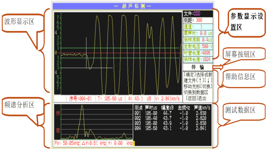
图 9.1 超声检测主界面
