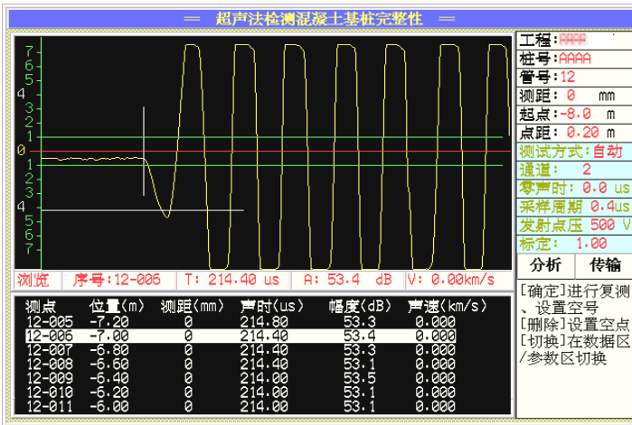
图 2.9 单通道测试界面
