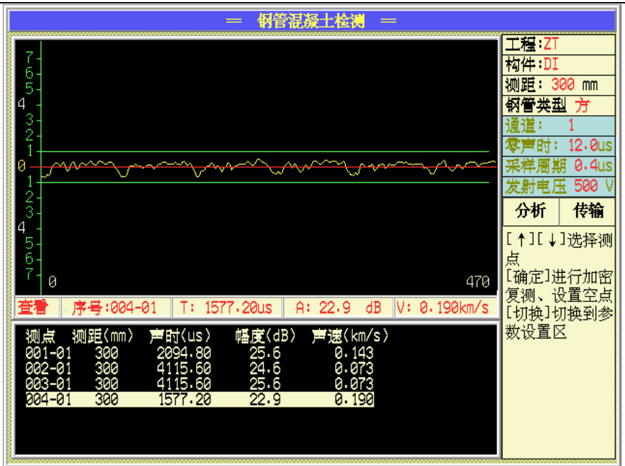
图 7.7 方管测试界面
