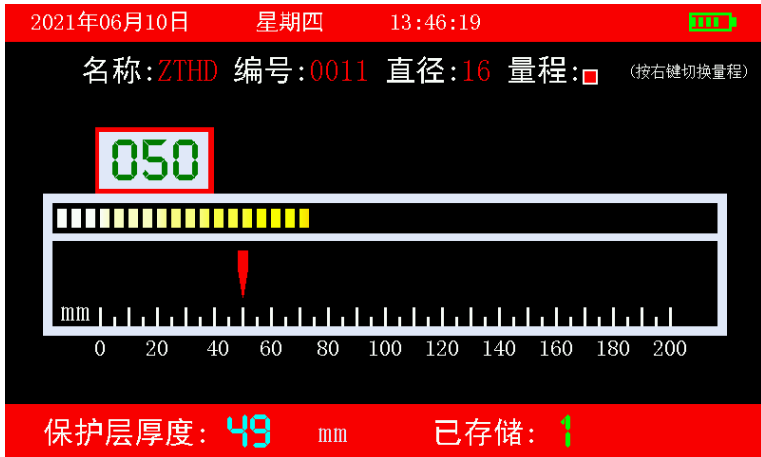
图 3.5 单点测试-厚度测试
